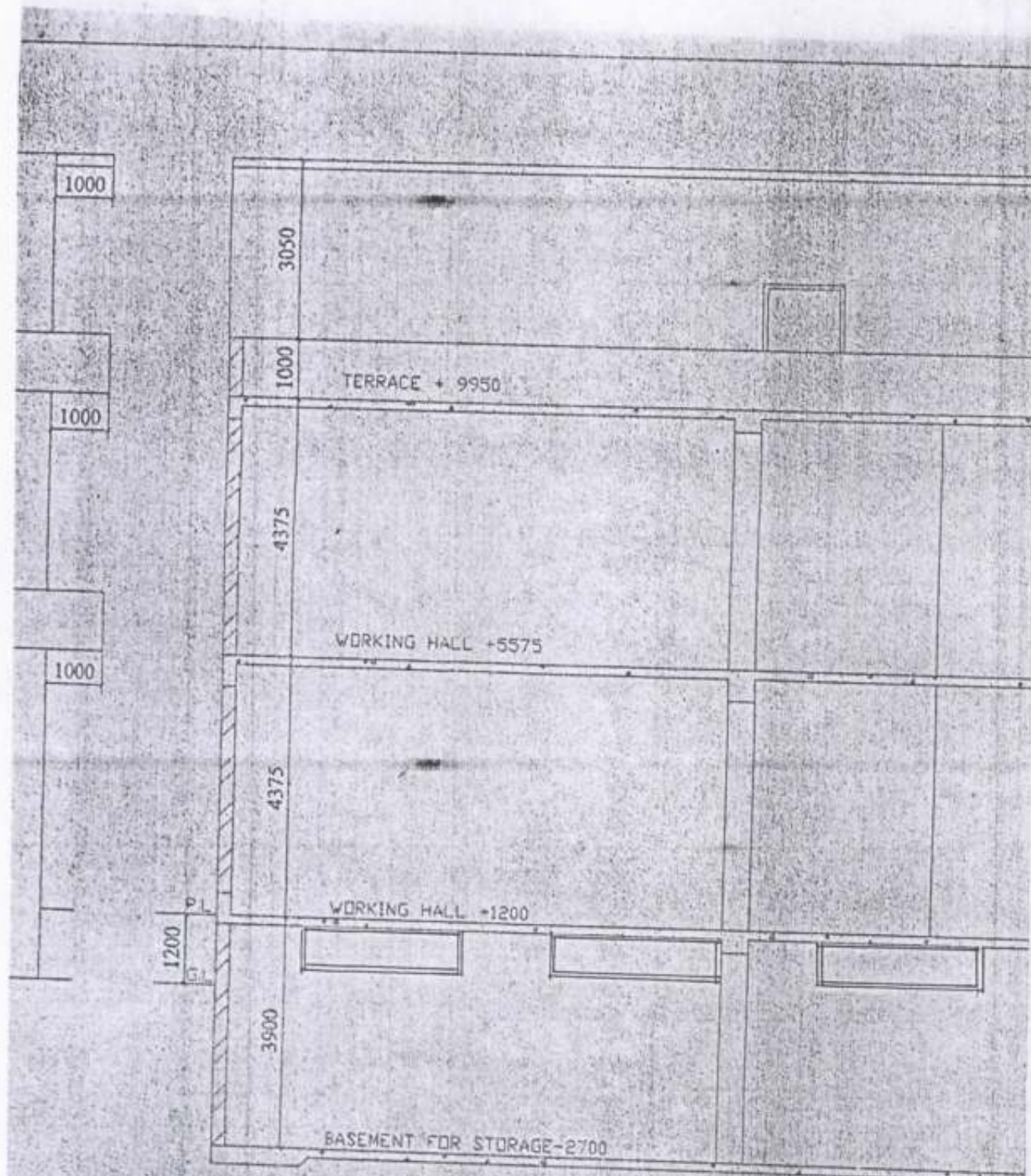
SECTION A-A
