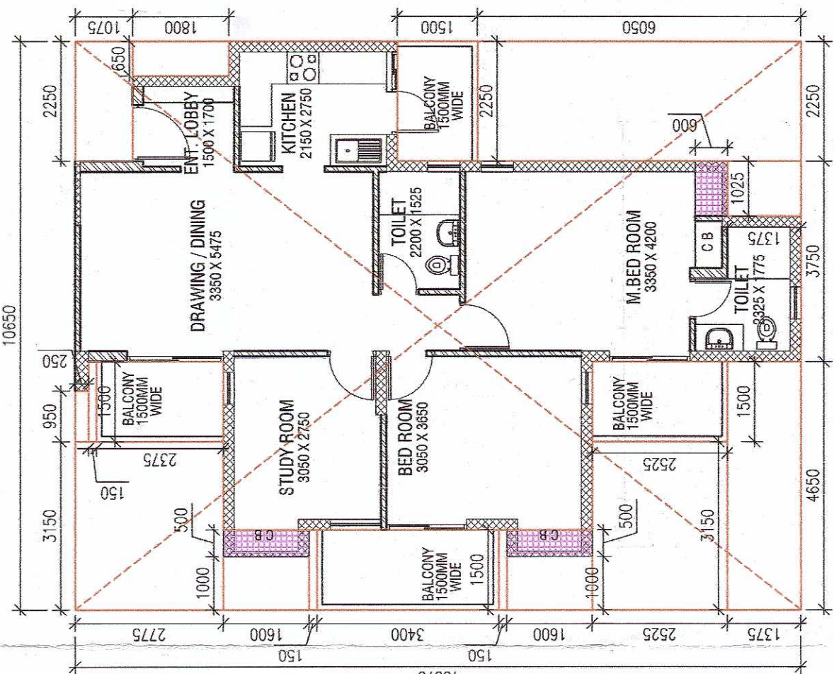
UNIT TYPE - 2a : 3 BED ROOM +2 TOILET
