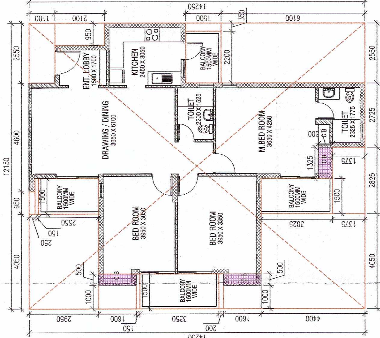
UNIT TYPE - 3 : 3 BED ROOM +2 TOILET
