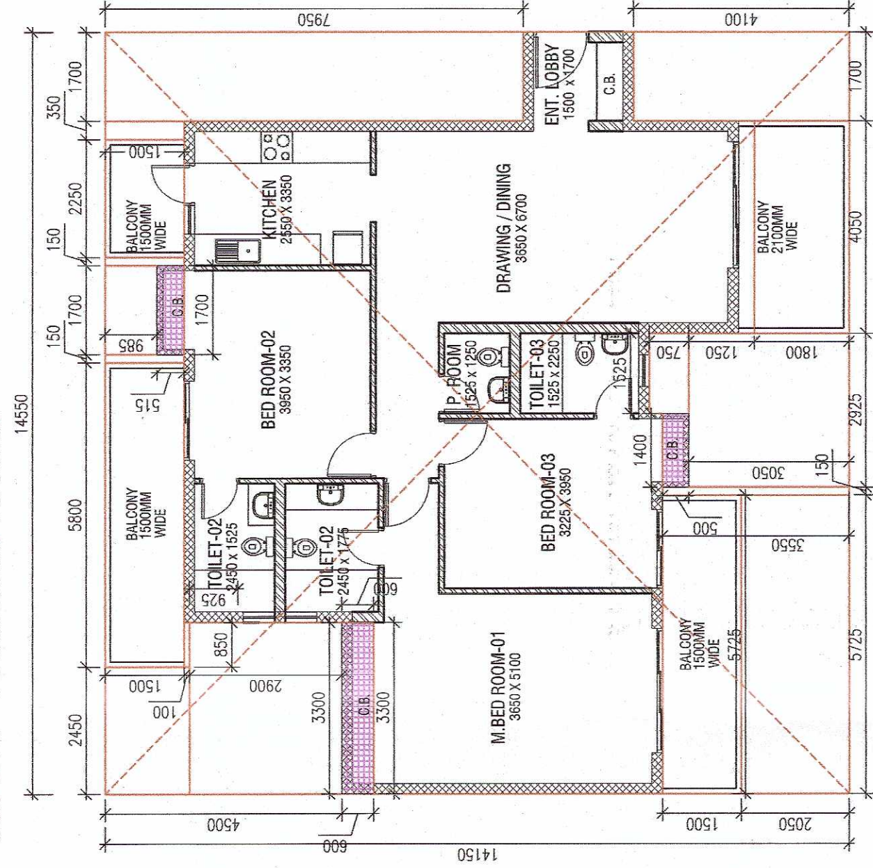
UNIT TYPE - 4 : 3 BED ROOM +3 TOILET
