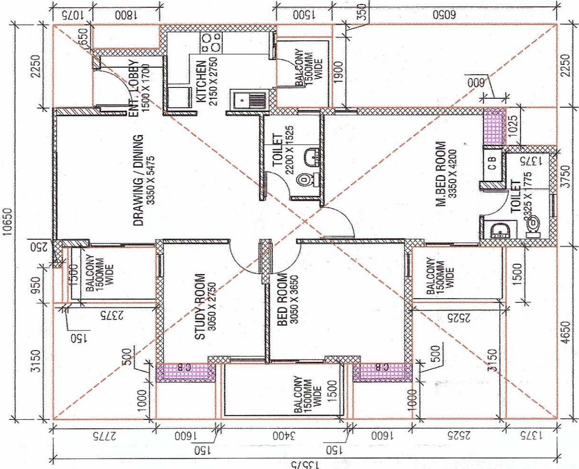
UNIT TYPE - 2 : 3 BED ROOM +2 TOILET
