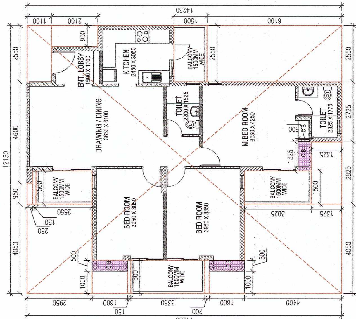
UNIT TYPE - 3a : 3 BED ROOM +2 TOILET
