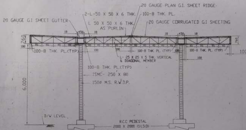
SECTION OF CANOPY SCALE - N.T.S.
