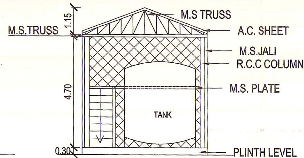
SECTION DD
