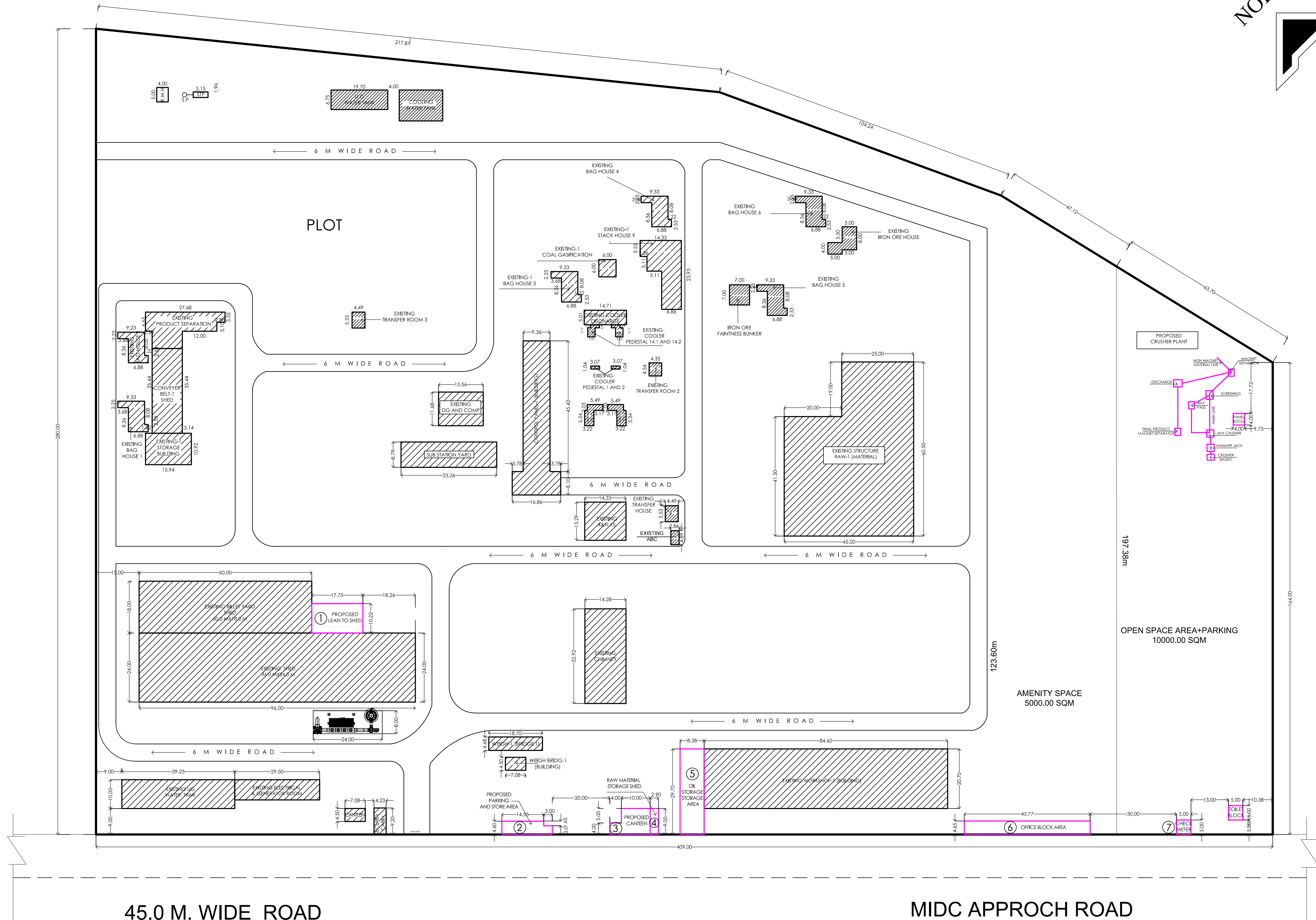
SITE PLAN ( 1:100)
