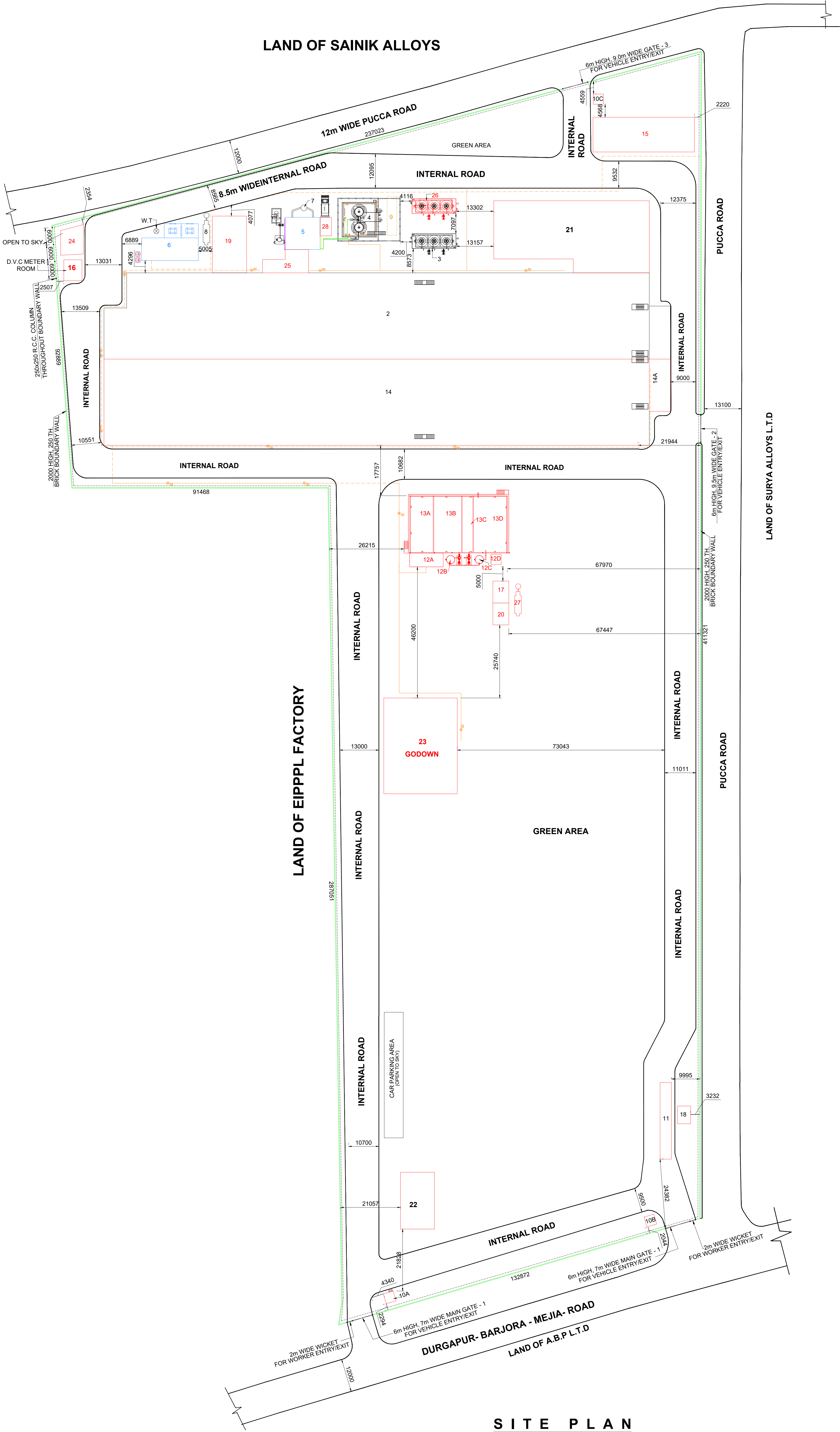
S I T E P L A N
